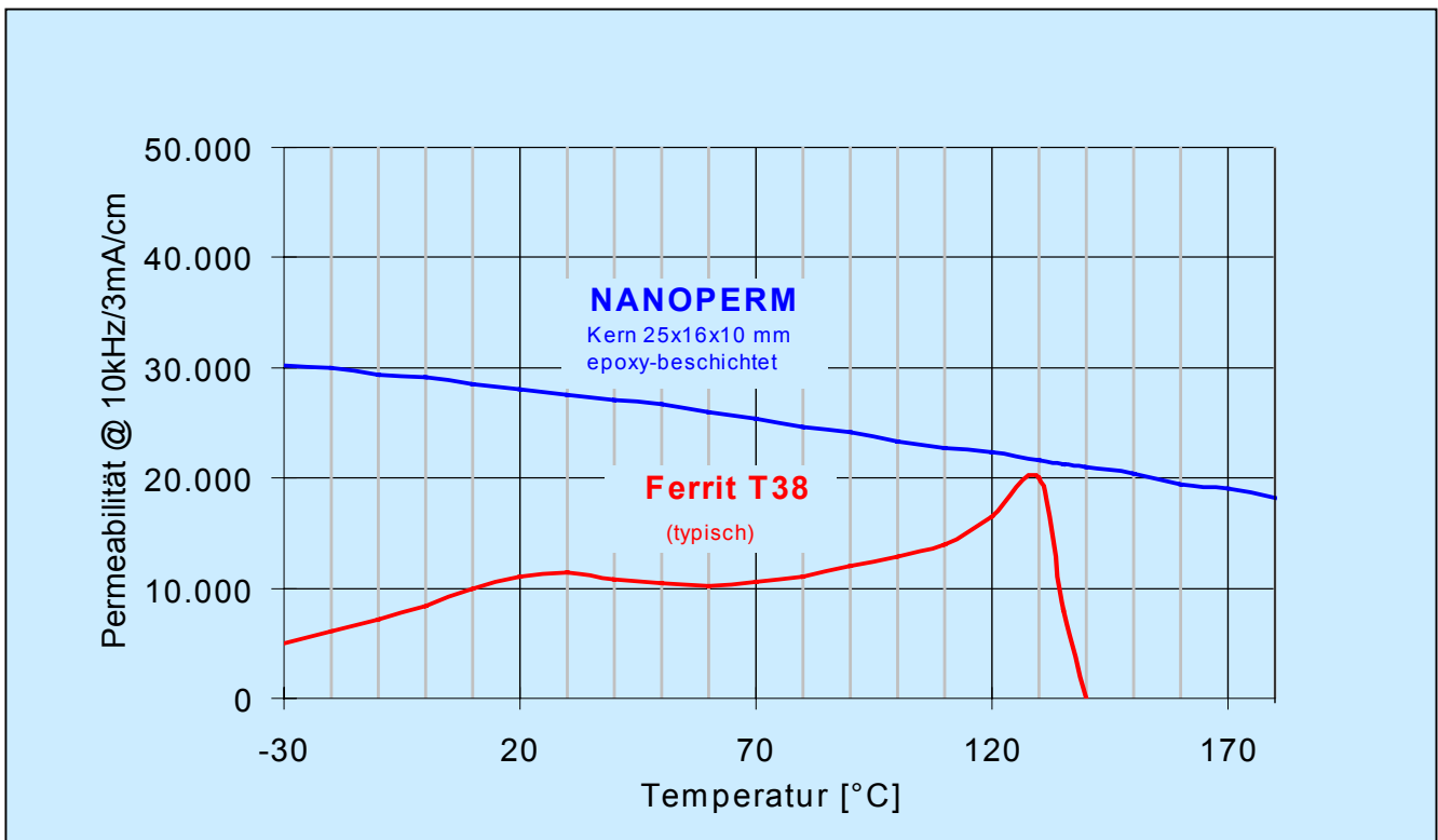
Permeabilität über die Temperatur
