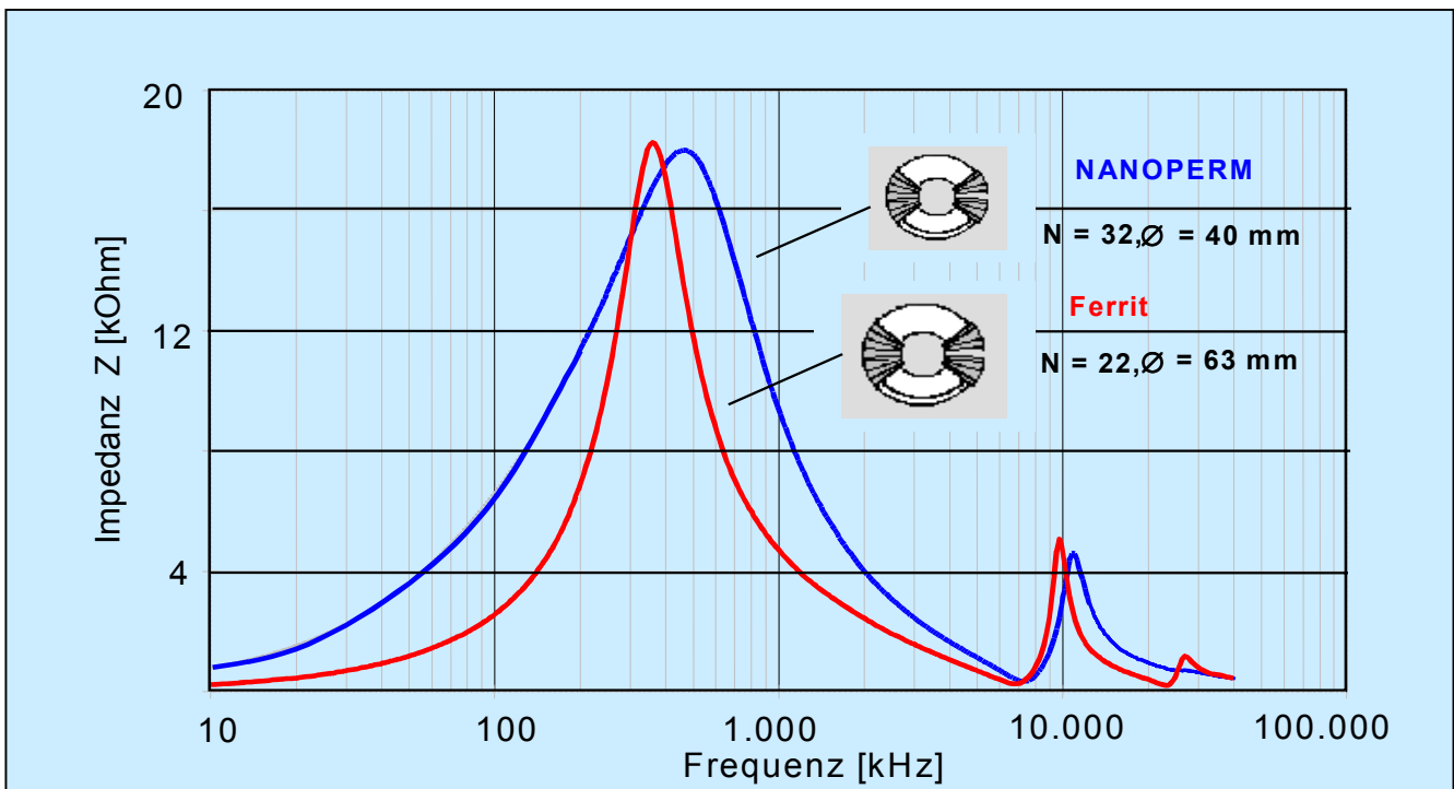
Einfügungsdämpfungsmessung - Gleicher Impedanzverlauf bei geringerem Bauvolumen
