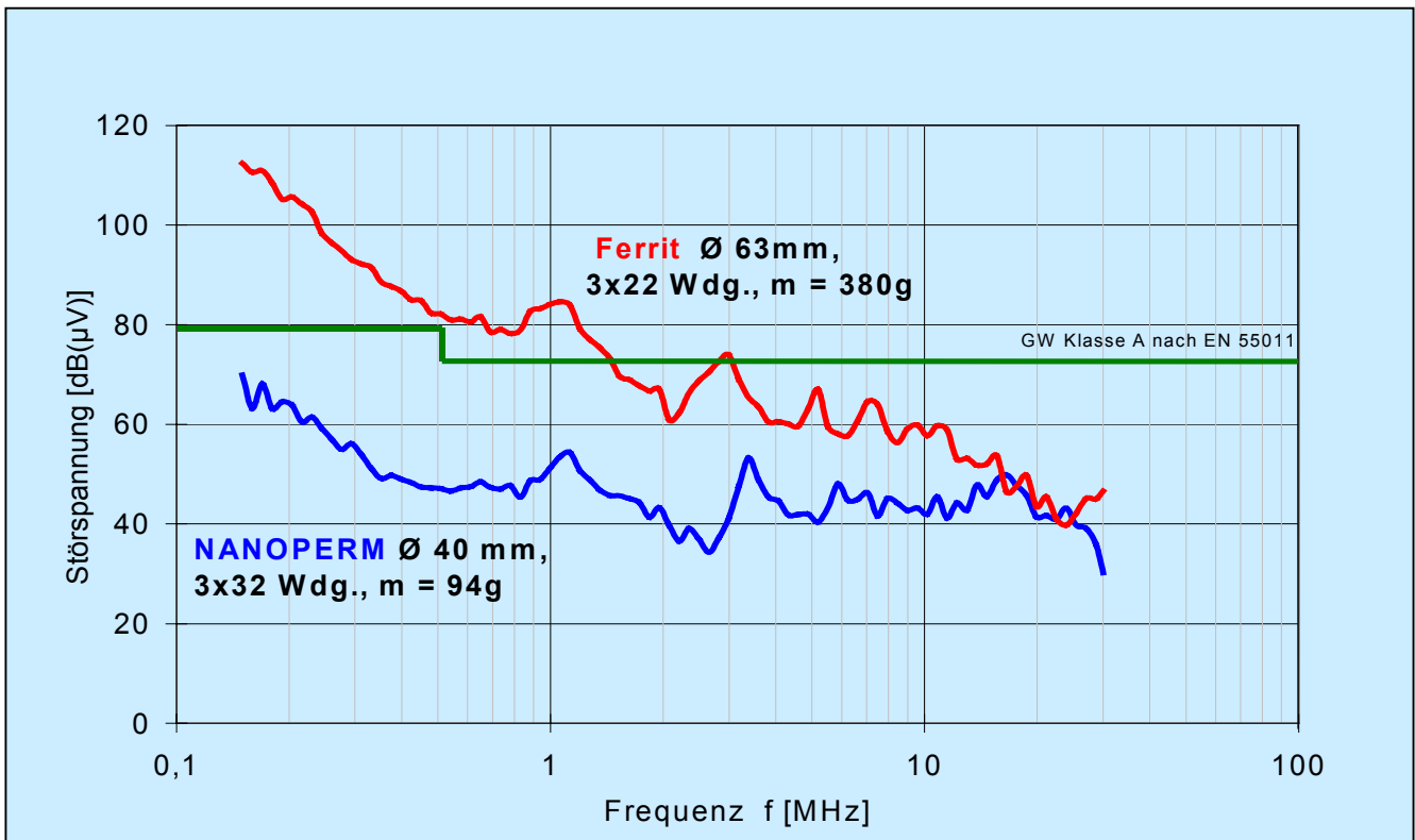
Funktörspannungsmessung – Bessere Entstörung bei geringerem Bauvolumen
